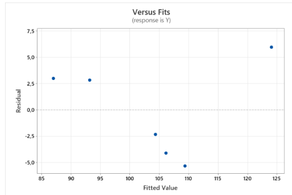
Gambar 3. Uji Heteroskedastisitas
