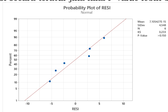
Gambar 2. Uji Normalitas
